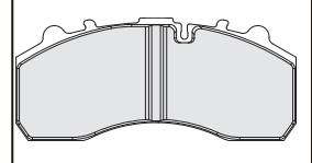
DCV1914FE (248x108x30mm) 29196
