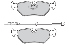
FD6897V BRE 23921 110 x 49.9 x 20.1mm
