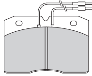
FD6320V BRE 29041 110 x 73 x 18.3mm
